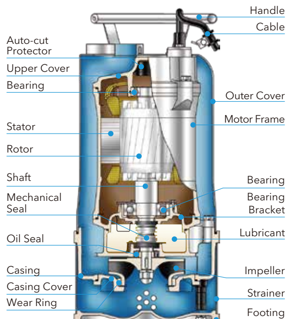
Close Impeller
